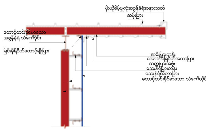
တိုးချဲ့အခုံးပါဝင်သော အစွန်းအနားပုံစံ
