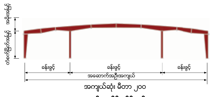
အကျယ်ဆုံး မီတာ ၂၀၀ အလယ် ၂ တိုင် ဖရိန်စနစ်-၂
