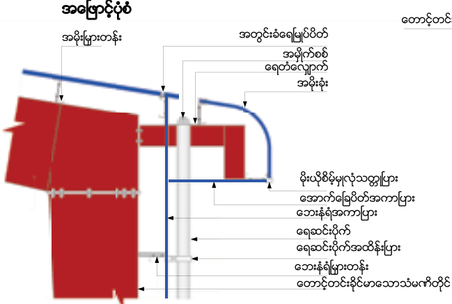
အောက်ခြေပိတ်အကာပြား နှင့် ရေတံလျှောက် ပါဝင်သော တံစက်မြိတ်အခုံးပုံစံ
