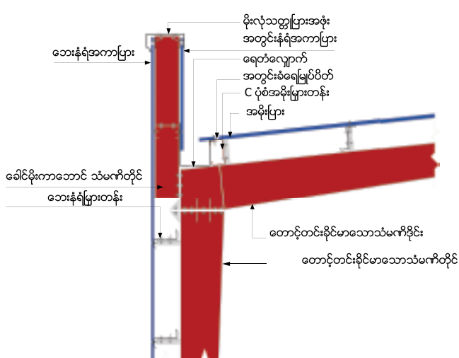
ခေါင်းမိုးကာဘောင် အပြောင့်ပုံစံ
