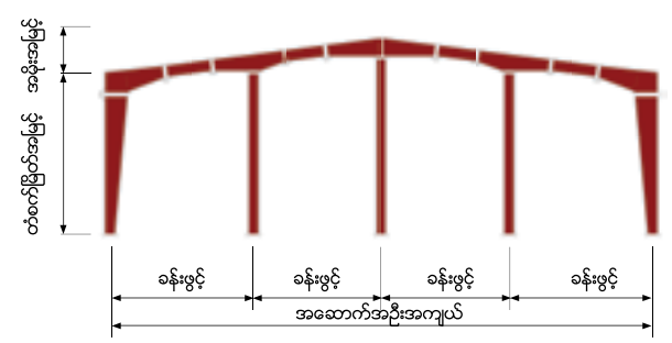
အကျယ်ဆုံး မီတာ ၄၀၀ အလယ် ၃ တိုင် ဖရိန်စနစ်
