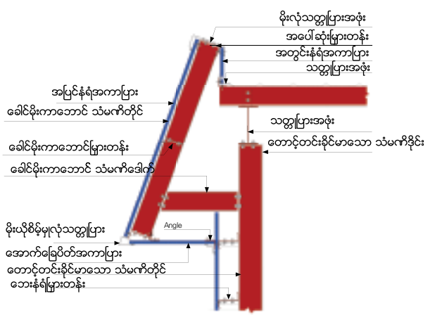
ခေါင်းမိုးကာဘောင် အစောင်းပုံစံ
