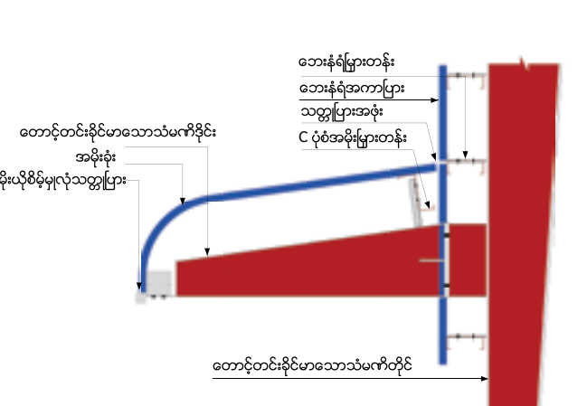
နေကာအခုံးပုံစံ
