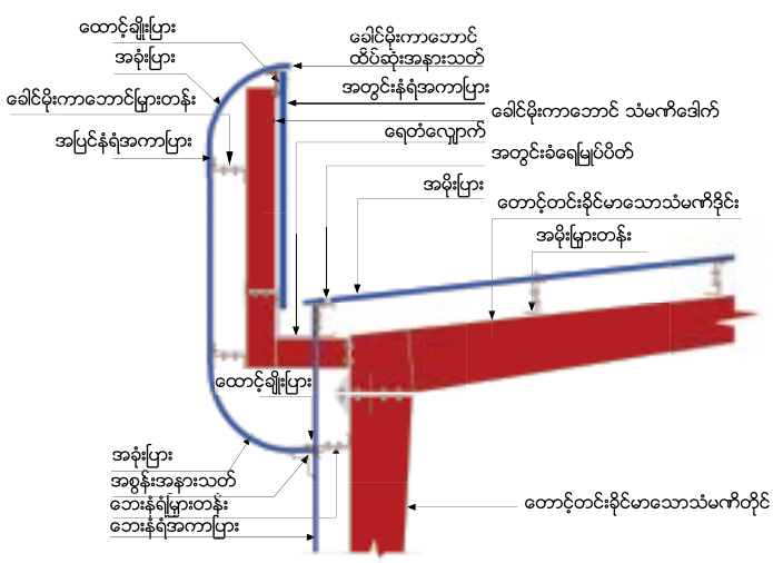
ခေါင်းမိုးကာဘောင် အခုံးပုံစံ
