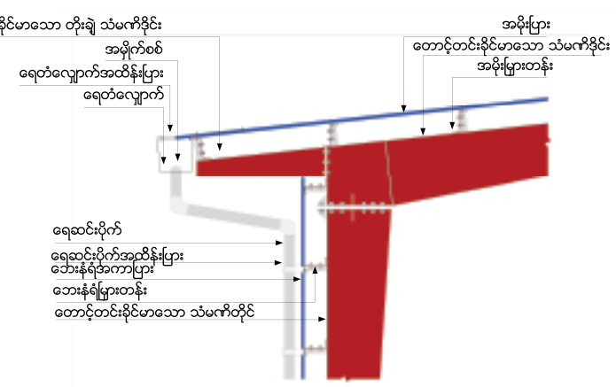
တိုးချဲ့အခုံးပါဝင်သော တံစက်မြိတ်ပုံစံ
