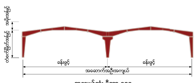
အကျယ်ဆုံး မီတာ ၁၅၀ ဆင့်ပွားဖရိန်စနစ်-၁ (အလယ်တိုင်ပျောက်အမိုးနှစ်ခုဆက်)
