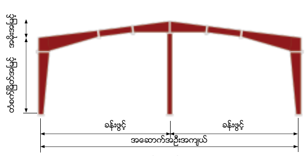
အကျယ်ဆုံး မီတာ ၁၅၀ အလယ် ၁ တိုင် ဖရိန်စနစ်
