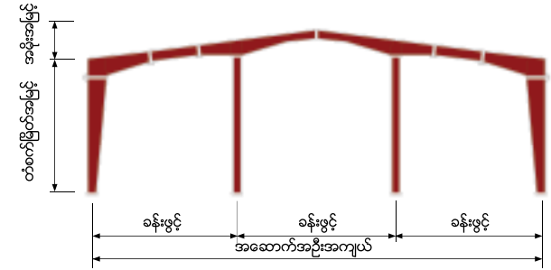
အကျယ်ဆုံး မီတာ ၂၀၀ အလယ် ၂ တိုင် ဖရိန်စနစ်
