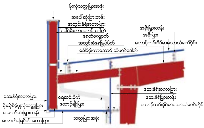
အောက်ခြေပိတ်အကာပြား နှင့် ရေတံလျှောက်ပါဝင်သော ခေါင်းမိုးကာဘောင်
