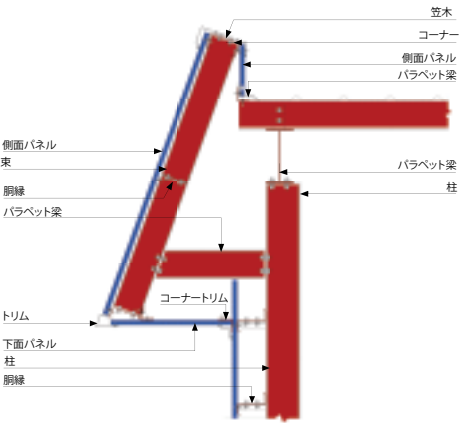
斜パラペット
