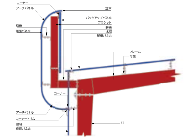
アーチパラペット
