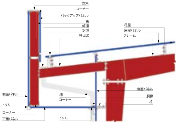
垂壁付パラペット
